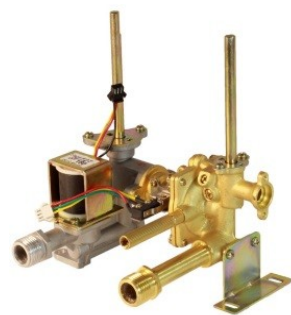
Газоводяной блок (10 л) "Vektor", "Нева" 4610
