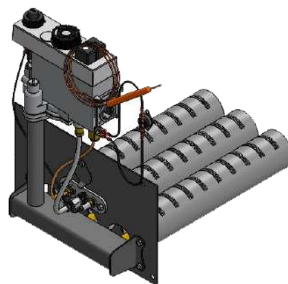
Правый подвод газа
