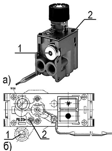
Рисунок19. Узлы регулировки:
