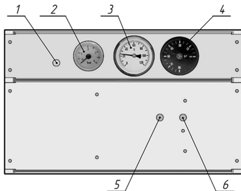
Рис. 14 Приборная панель
