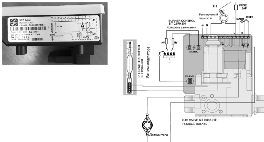
Рис. 13 Схема подключений
