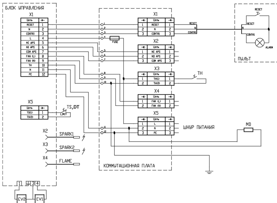
Рис. 15 Схема подключений с коммутационной платой
