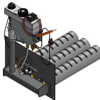
Правый подвод газа
