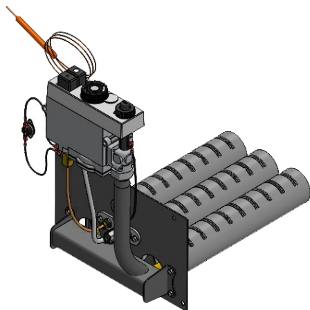
Левый подвод газа
